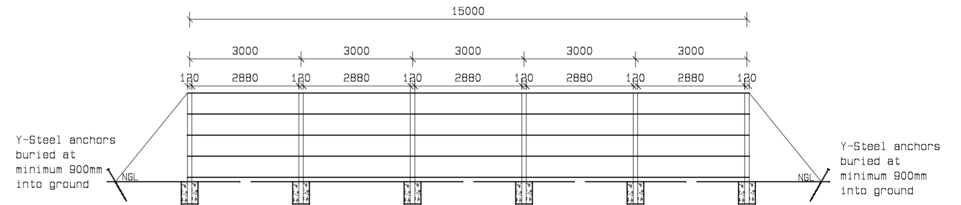
REAR ELEVATION Scale: 1:100
